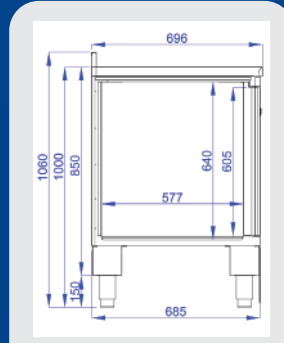
Ölçü Detayları Dimension Details
