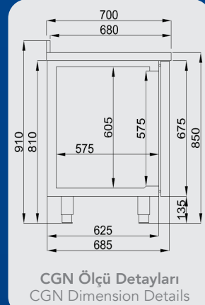
CSN Ölçü Detayları CSN Dimension Details
