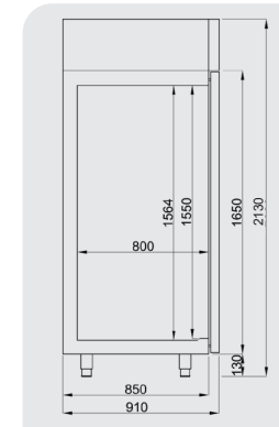
Ölçü Detayları Dimension Details
