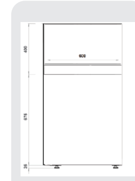
Ölçü Detayları Dimension Details
