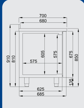
CGN Ölçü Detayları CGN Dimension Details
