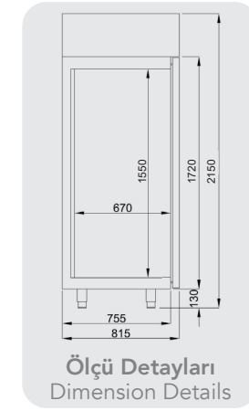
85 mm İzolasyon Kalınlığı 85 mm thickness
