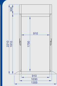
Ölçü Detayları Dimension Details
