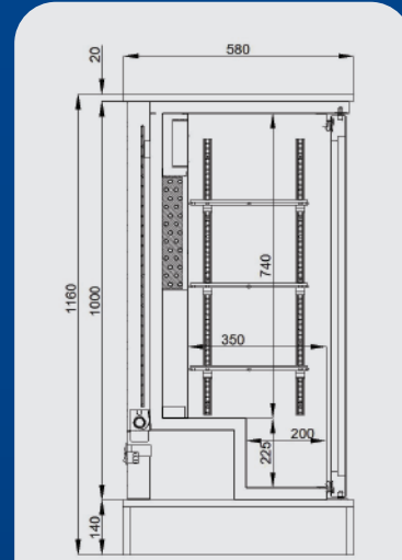
Ölçü Detayları Dimension Details
