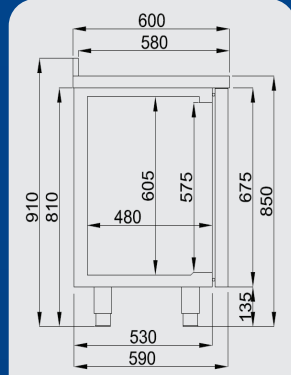
CSN Ölçü Detayları CSN Dimension Details
